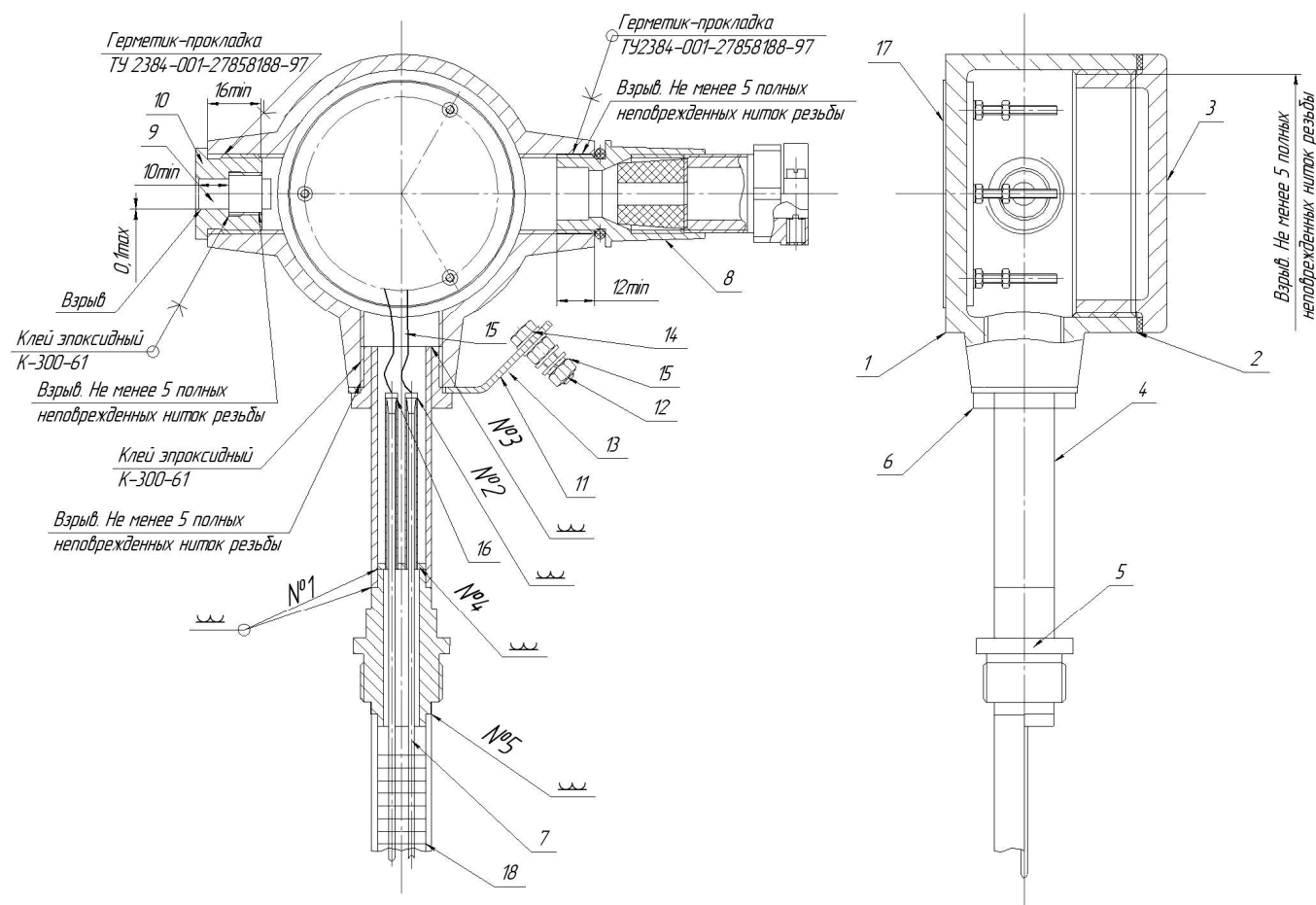
Рис.3. Средства взрывозащиты прибора
