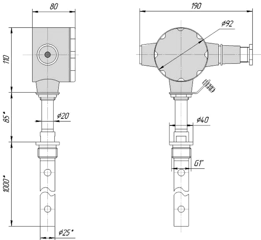
Рис. 2 Внешний вид прибора контроля уровня жидкости СЖУ-1-ВУ2.
