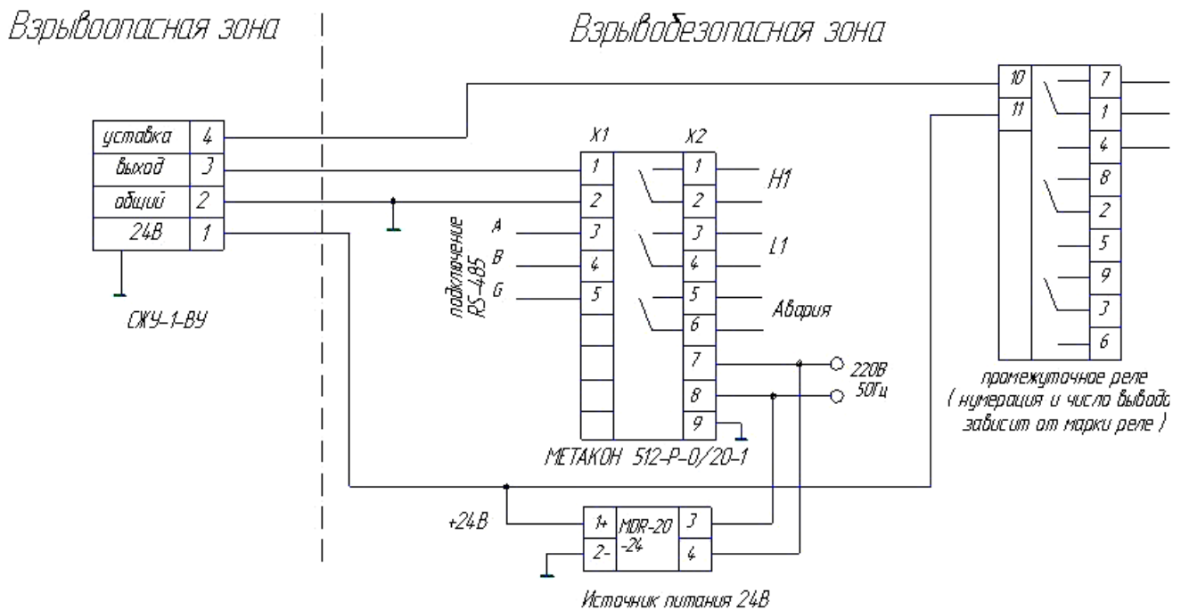
Рис.4. Схема подключения прибора по 4-х проводной схеме
