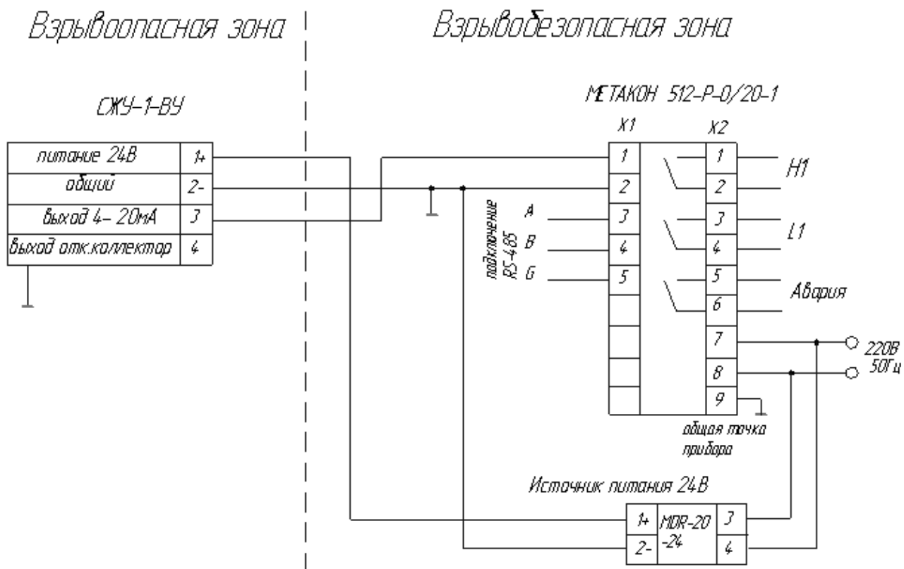
Рис.3. Схема подключения прибора
